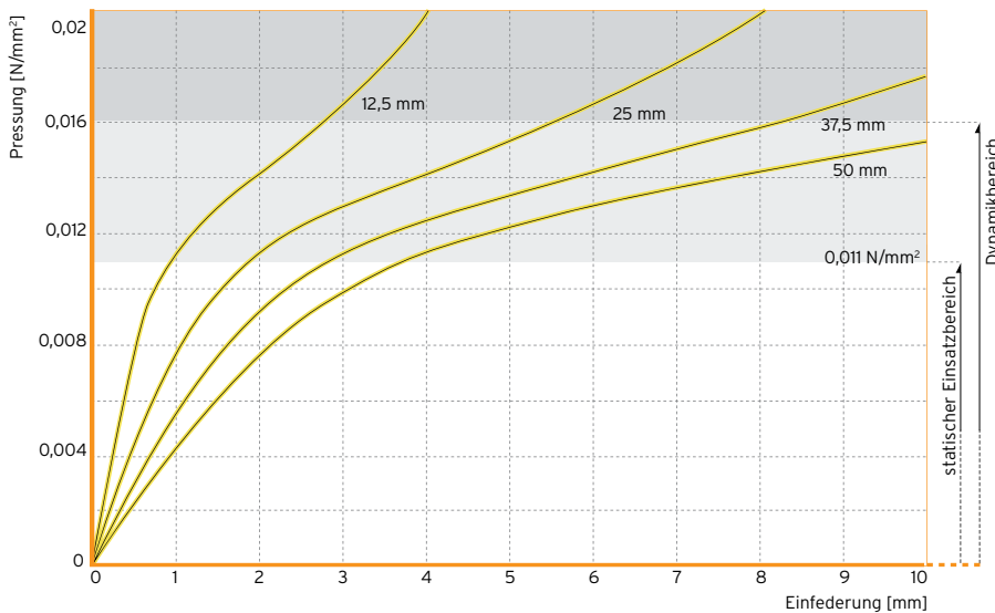
Abb. 1: Quasistatische Federkennlinie mit einer Belastungsgeschwindigkeit von 0,0011 \text{ N/mm}^2/\text{s}
