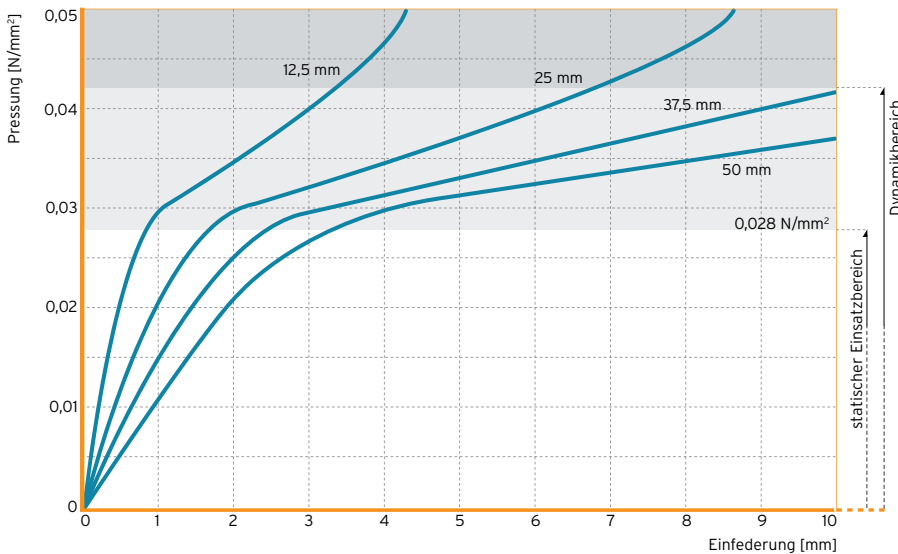
Abb. 1: Quasistatische Federkennlinie mit einer Belastungsgeschwindigkeit von 0,0028 N/mm 2 /s
