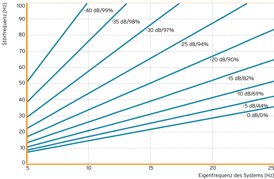
Abb. 4: Verminderung der Übertragung mechanischer Schwingungen durch den Einbau einer elastischen Lagerung aus Sylomer SR 28 auf starrem Untergrund
